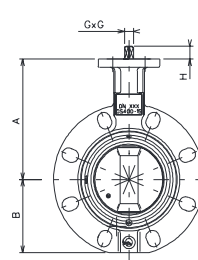
kołnierz pojedynczy
