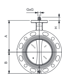
dwa kołnierze
